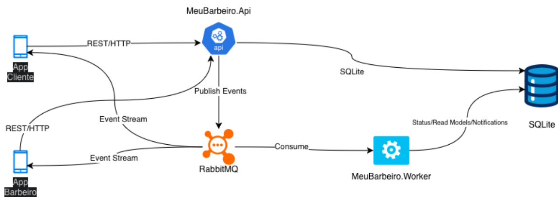
Figura 1 – Arquitetura inicial do sistema MeuBarbeiro.
